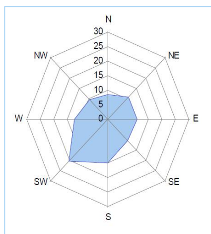
Joonis 10. Aastane tuuleroos Pärnu MHJ andmeil (1971-2000)
