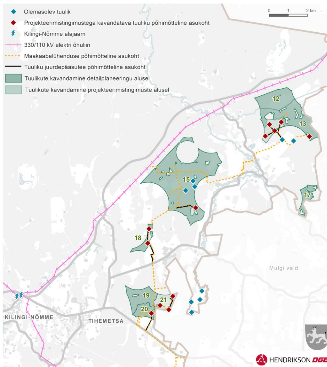
Skeem 5.4.5.3-1 Tuuleenergeetika alad, olemasolevate tuulikute ning kavandatavate tuulikute, juurdepääsuteede ja maakaabelliinide põhimõttelised asukohad.
